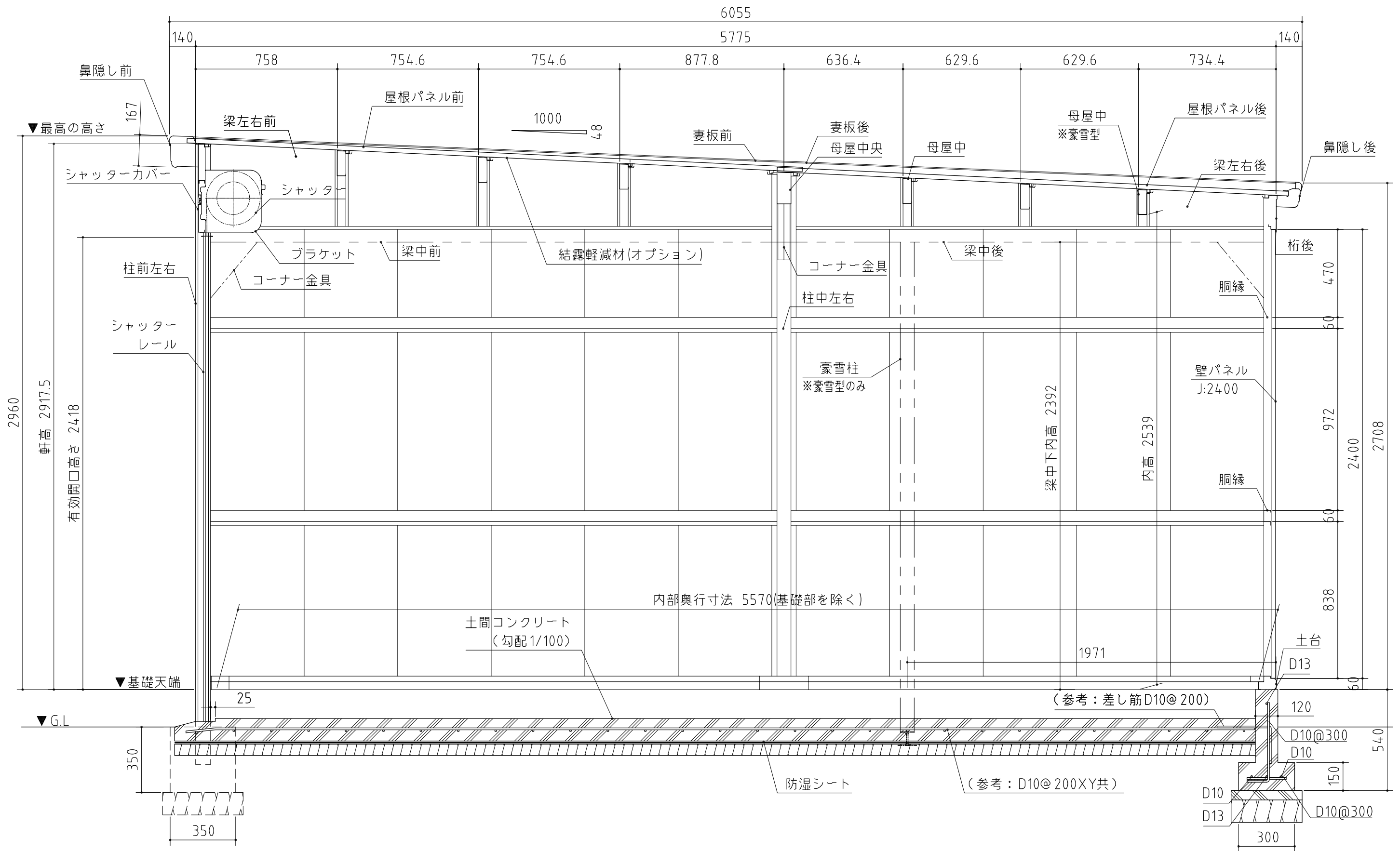
断面図 (側面) (縮尺) S=1/20 ~一般型・豪雪型~ 機種名 GRN-2657J・JL, 3157J・JL, 3657J・JL
